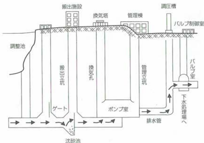
〔図2〕TARP 断面概念図
