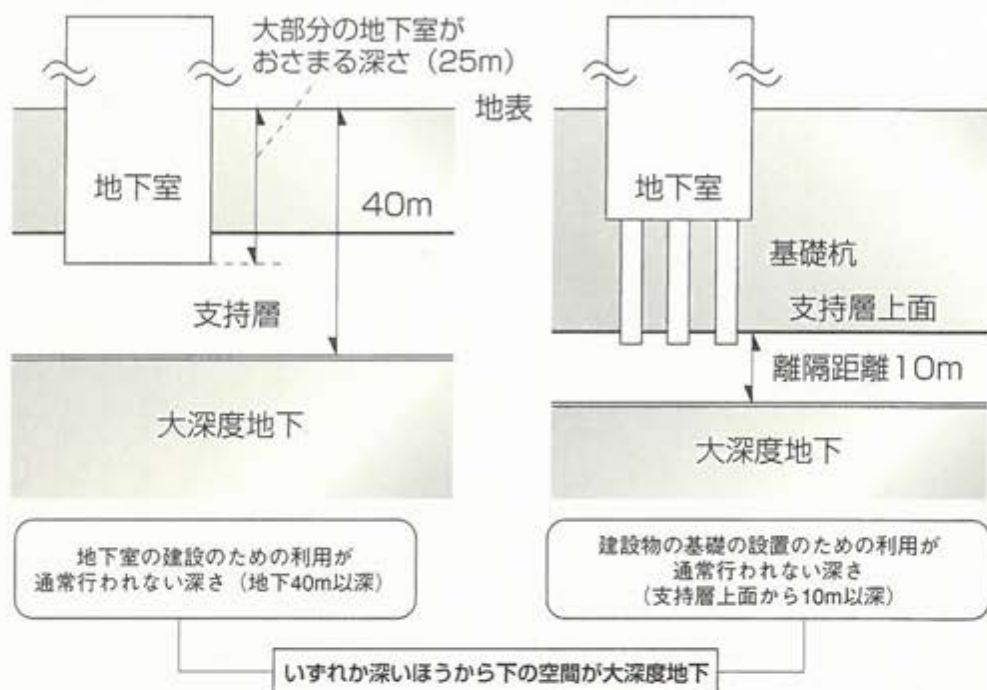
【図2】大深度地下の定義図
