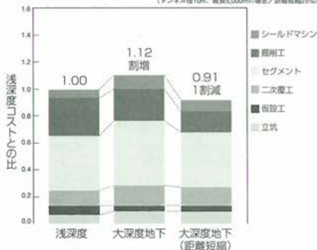
【図5】大深度地下利用に当たっての建設コスト試算
